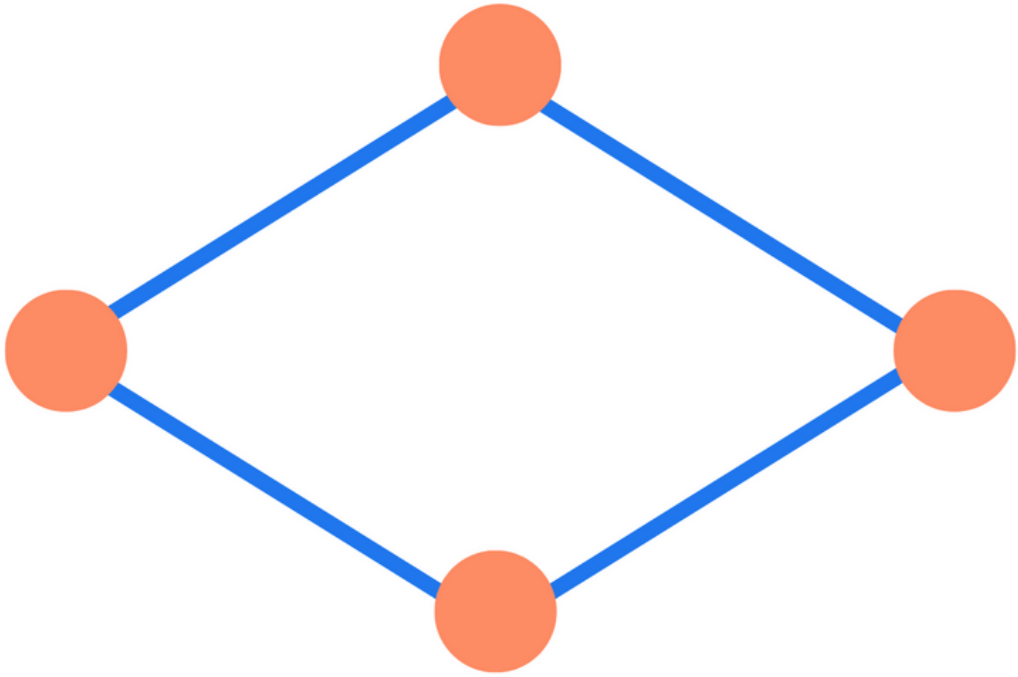
Diamond (마름모)
